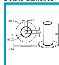
Detalle diámetros
